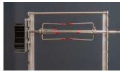
RÔTISSOIRE (montage uniquement sur stop-food Grill'Chic)
